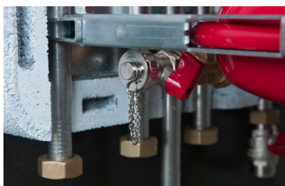
28. Påfyldningsventil (bundhane).
