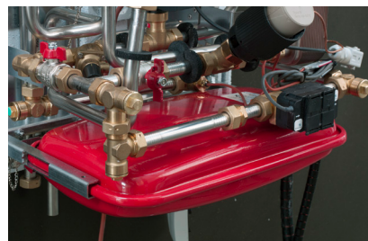
34. Trykexpansionsbeholder til at optage vandets udvidelse ved opvarmning.
