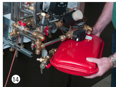
14. Udsiftning af ekspansionsbeholder sker ved at demontere vandforbindelsen til beholderen og trække beholderen ud af skinnerne, som fikserer beholderen.
